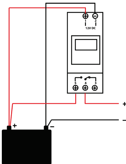
Normalement ouvert (NO)
