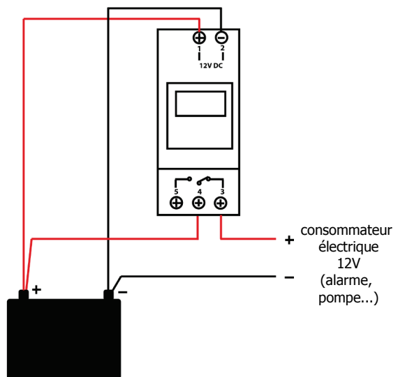
Normalement fermé (NF)
