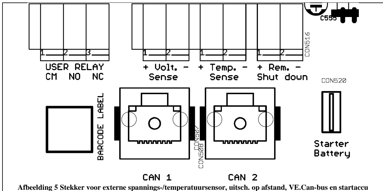
Afbeelding 5 Stekker voor externe spannings-/temperatuursensor, uitsch. op afstand, VE.Can-bus en startaccu
