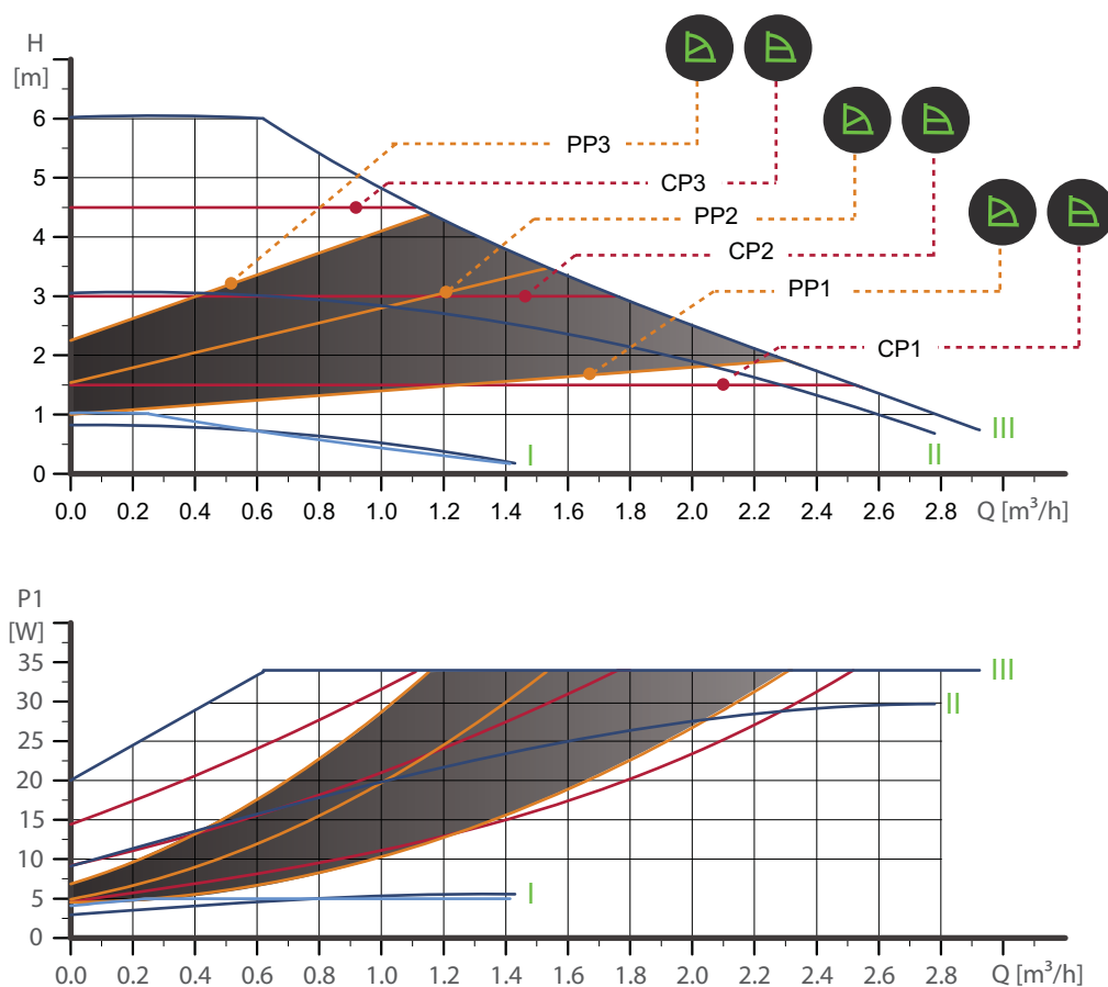
Fig. 35 ALPHA2 25-60 A
