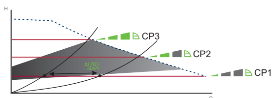
Fig. 19 Trois courbes/réglages de pression constante
