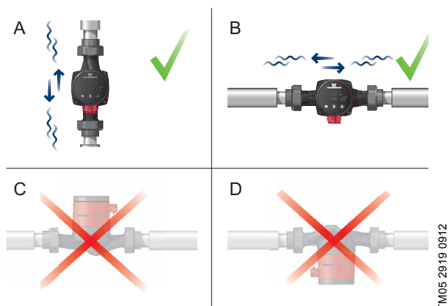
Fig. 6 Positions du coffret de commande
