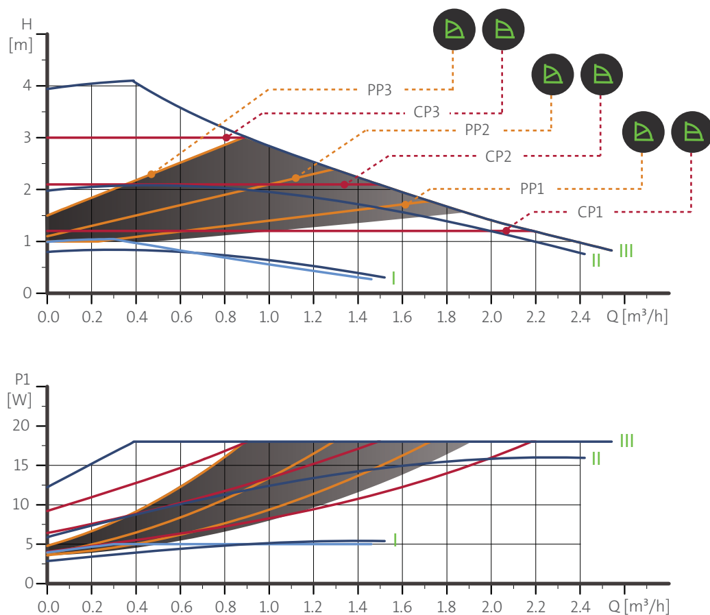
Fig. 31 ALPHA2 XX-40
