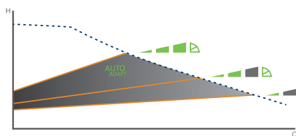
Fig. 14 Sélection du réglage du circulateur en fonction du type d'installation
