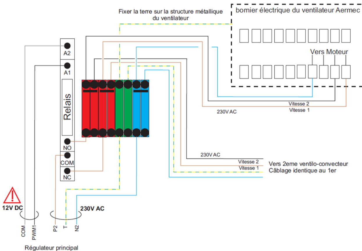
Schéma électrique pour ventilo-convecteur Aermec FCX double
