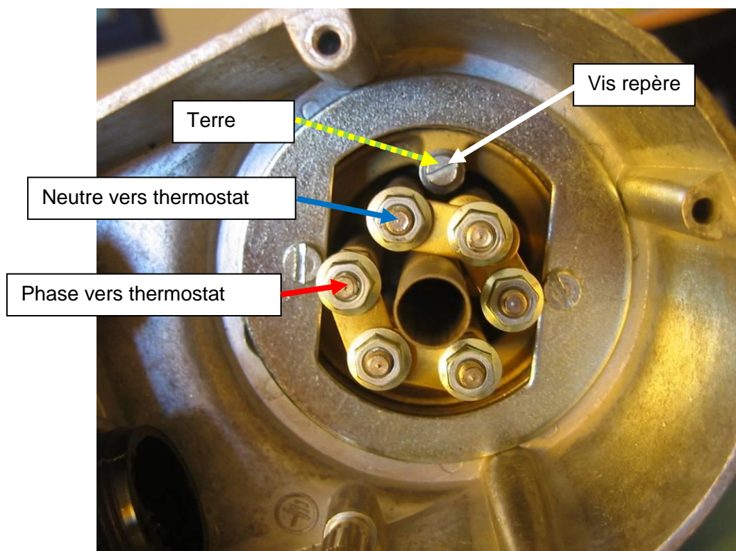
Bornes de la résistance électrique
