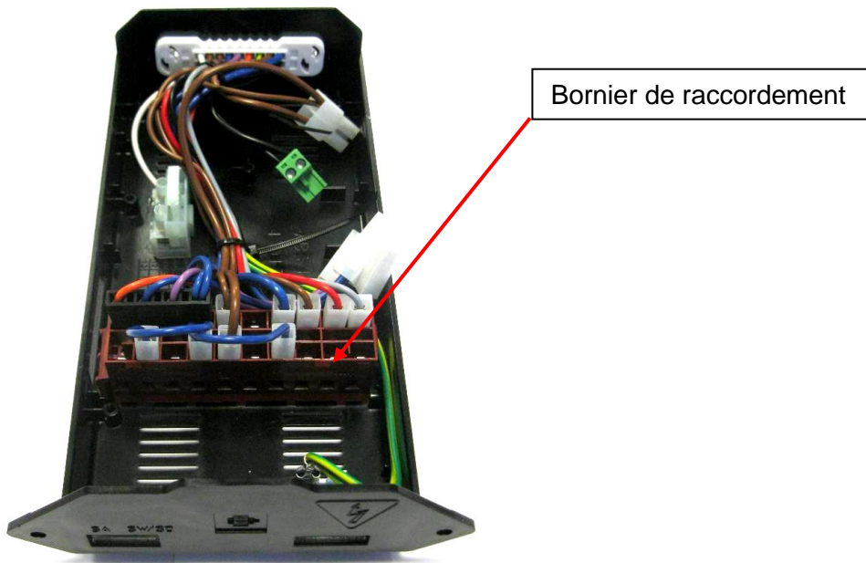
Boîtier électrique du ventilo-convecteur Aermec FCL
